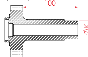
NIPLE ESTENDIDO (Face Plana)
